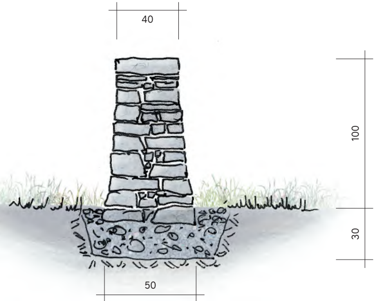
Mur de clôture
