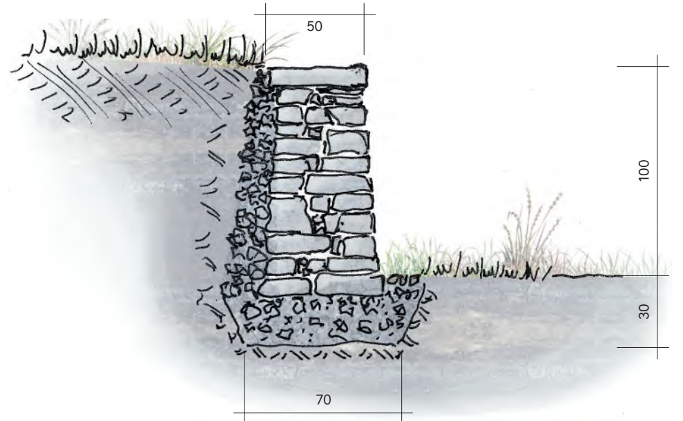
Mur de soutènement
