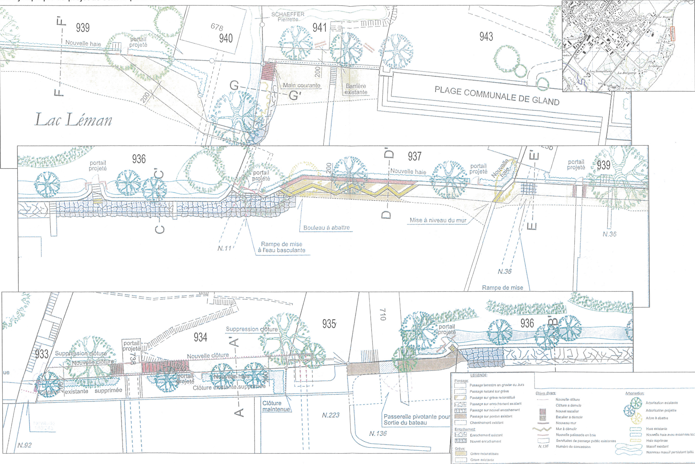
Plan synoptique du projet de sentier piétonnier
